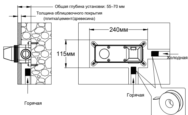
Встраиваемый корпус смесителя с блоком
